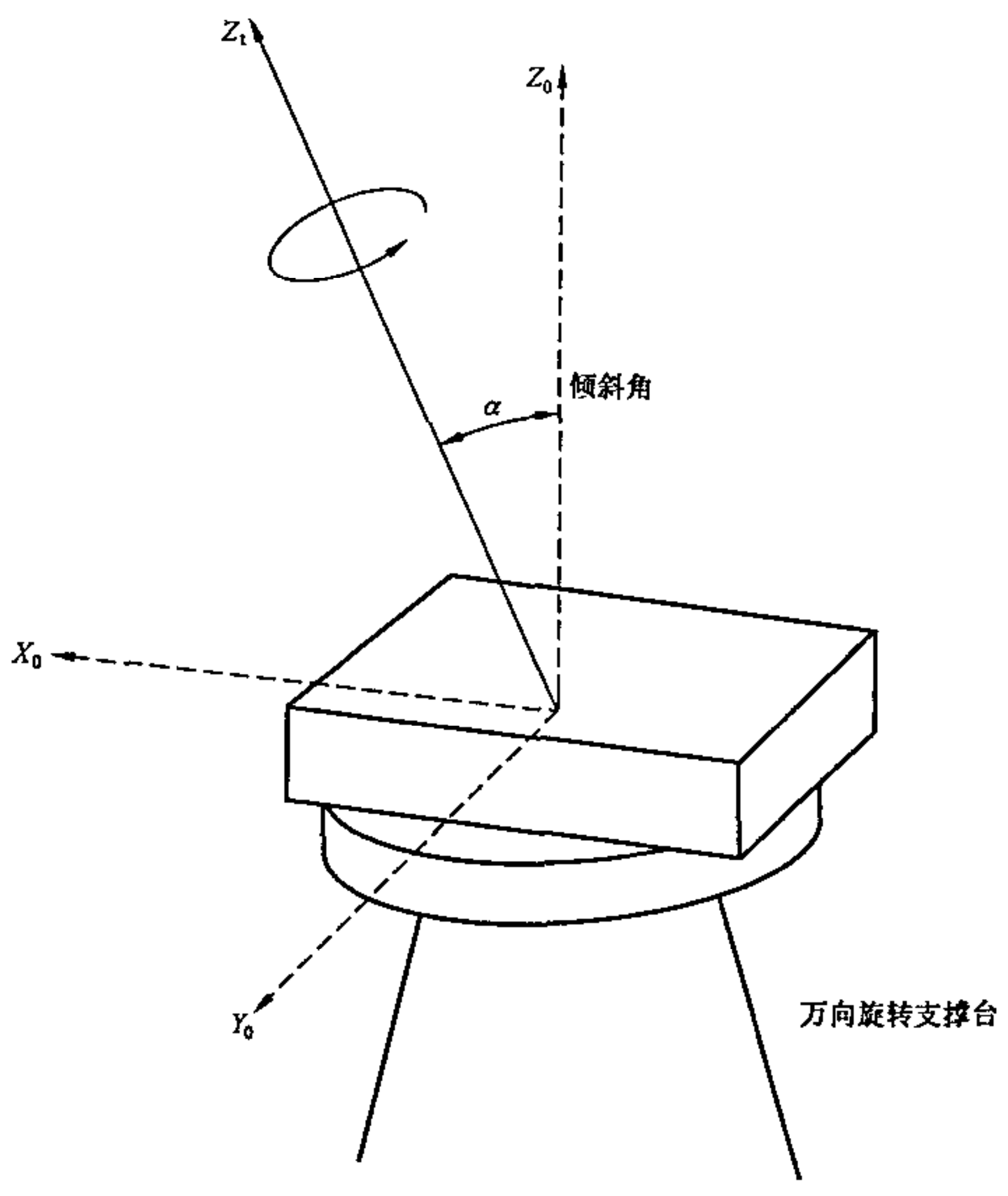
图 2 试验 Ra, 倾斜角和轴系的定义
